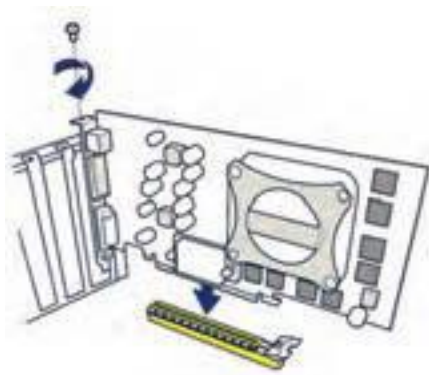
شکل ۴۷- نصب کارت گرافیک
